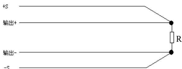
图 2.4 远端测量接线方法
