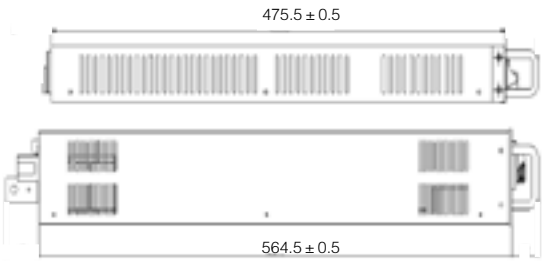
侧视图
